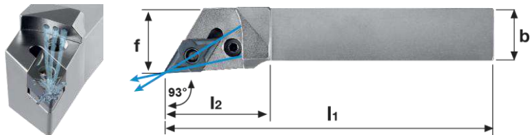
PDJNR/L Stelo in acciaio | Stahlschaft | Steelshank
