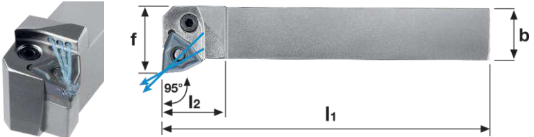
PVLNR/L Stelo in acciaio | Stahlschaft | Steelshank
