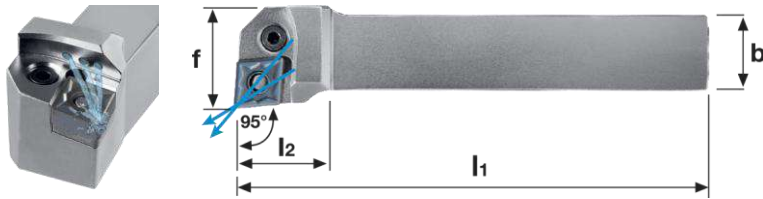
PCLNR/L Stelo in acciaio | Stahlschaft | Steelshank
